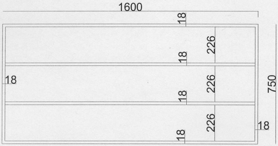
Widok front
