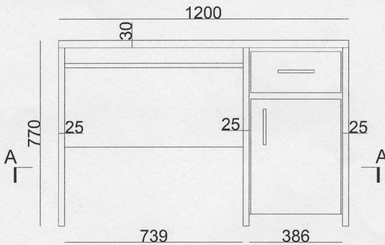
Widok front
