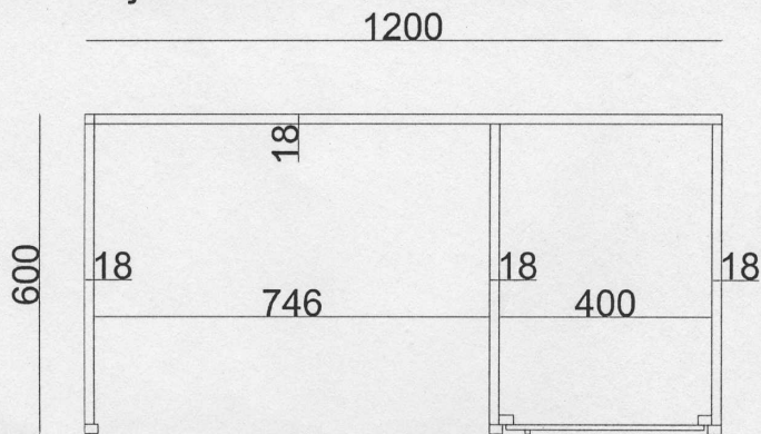
Przekrój A-A
