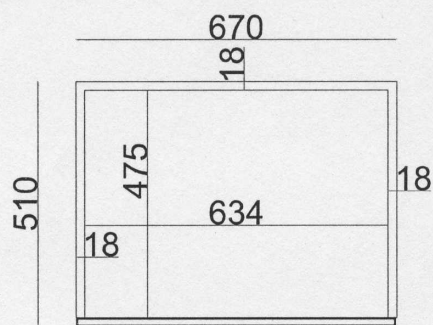
Przekrój A-A
