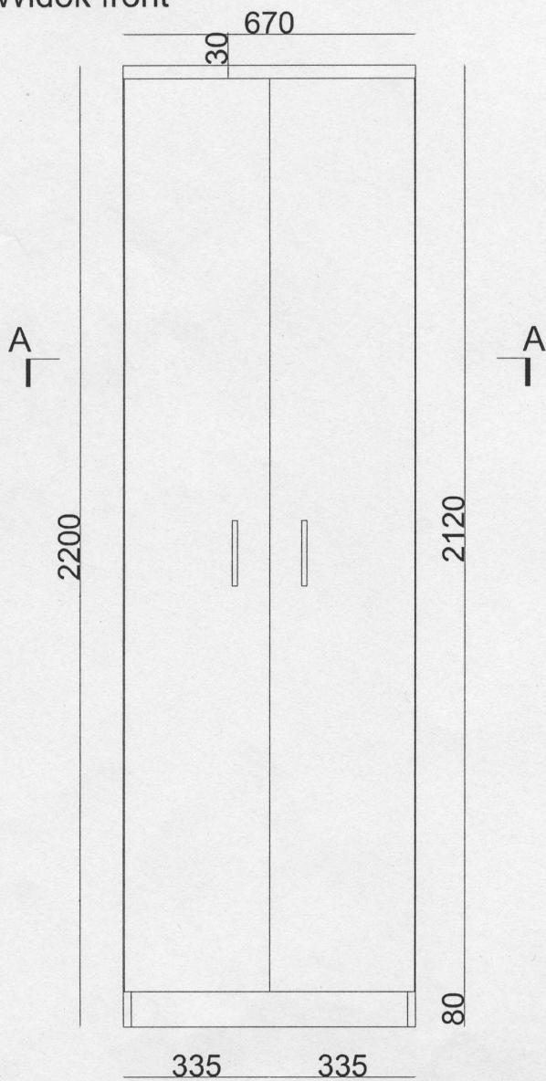
Widok front
