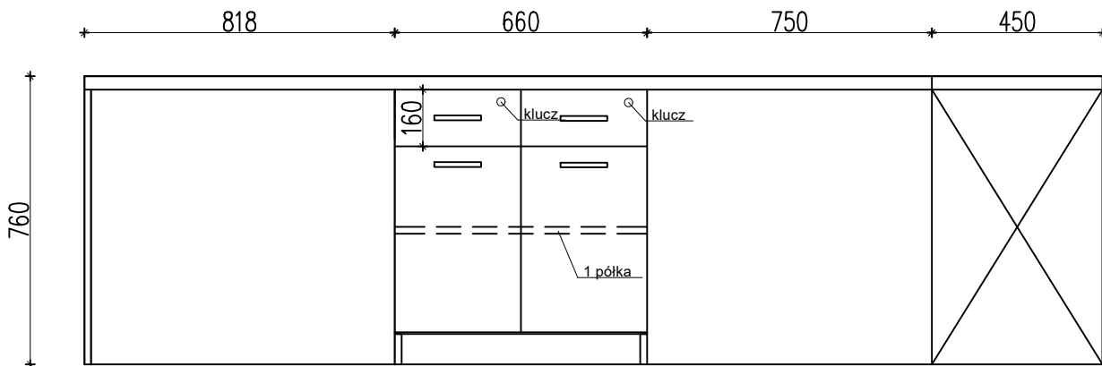
Widok front
