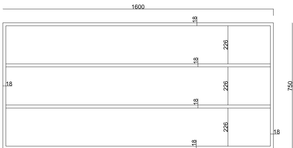
Widok front
